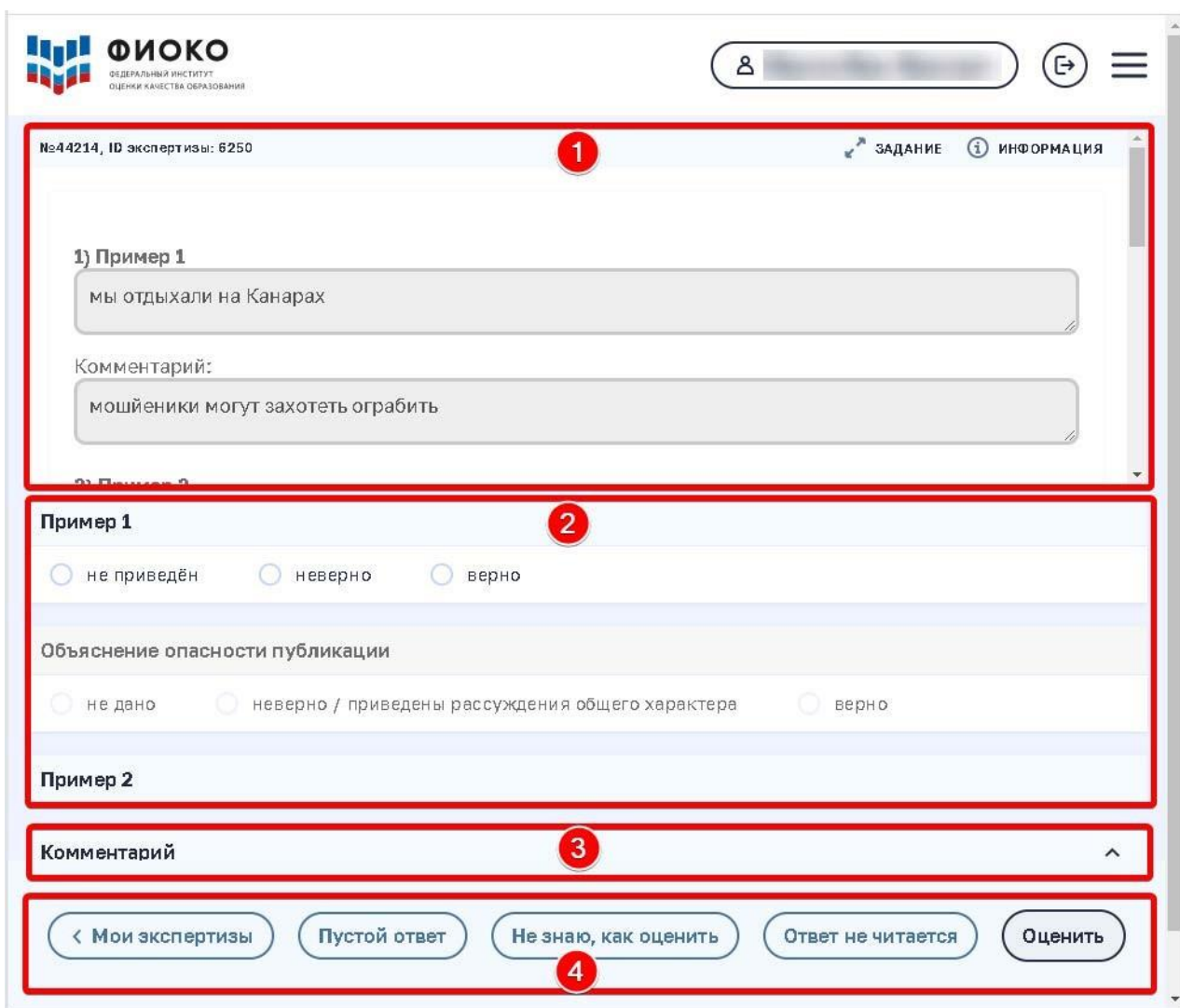
Рисунок 10. Элементы интерфейса для проведения экспертизы
